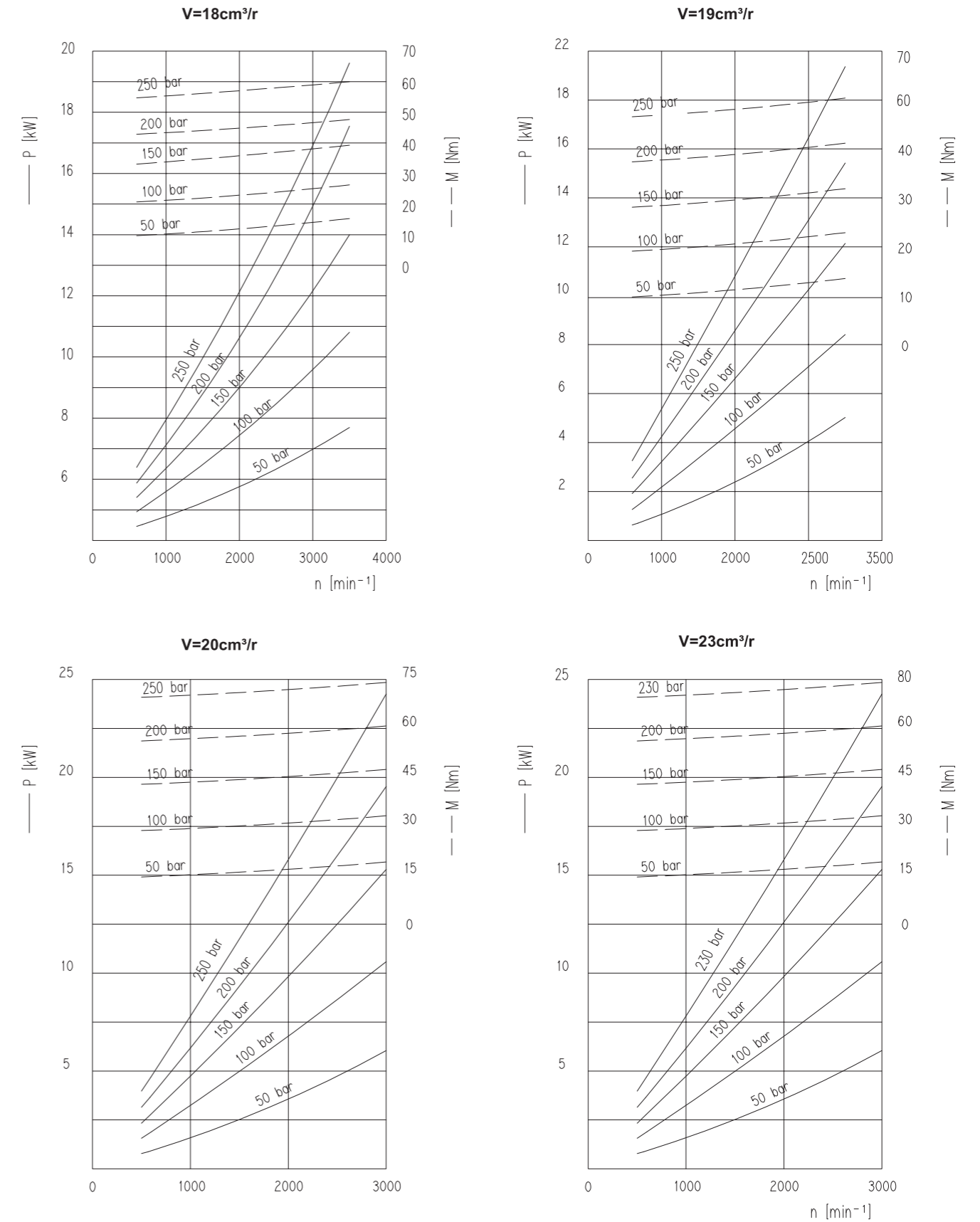
2.5系列功率性能曲线表/Group 2.5 Power Performance Curve Table
